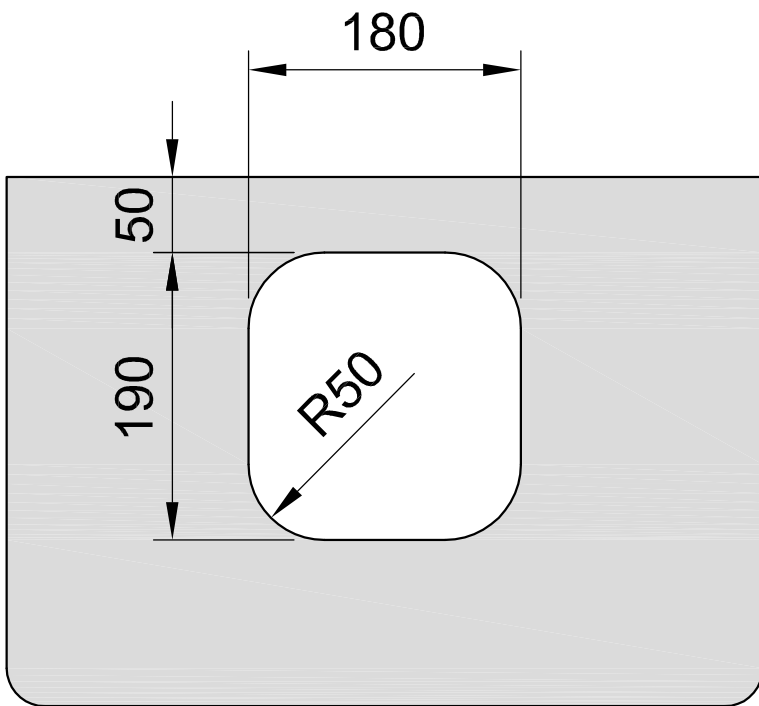
Detalle orificio encimera
